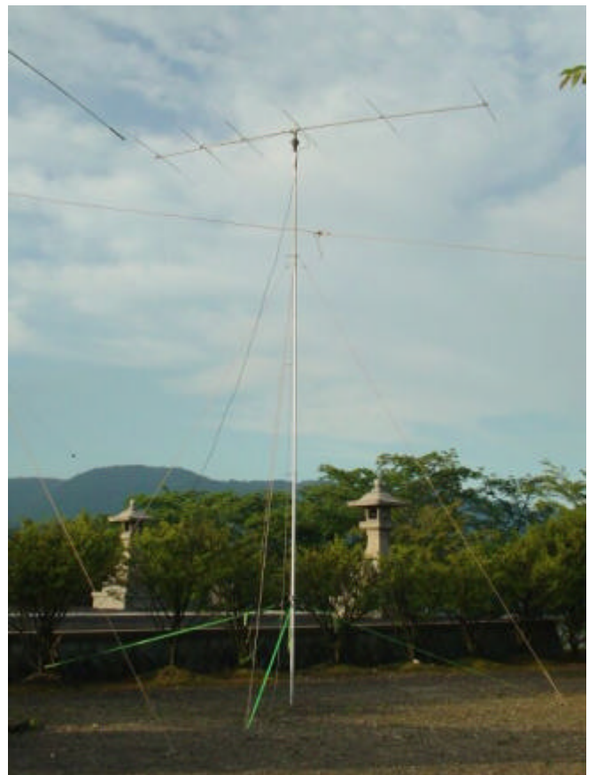
50MHz6エレのマストはラチェット機構付き荷締めバンドで垂直を出してからAnt・ローテータを載せ、一気にフルアップしています
